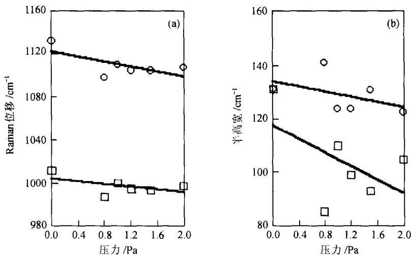
图 4 钠长石玻璃 1010 及 1100 cm -1 谱峰频率(a) 钠长石玻璃 1010 及 1100 cm -1 谱峰半高宽(b)与压力的关系
